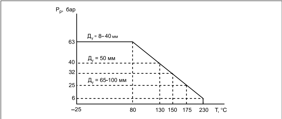
Зависимость рабочего давления от температуры перемещаемой среды
